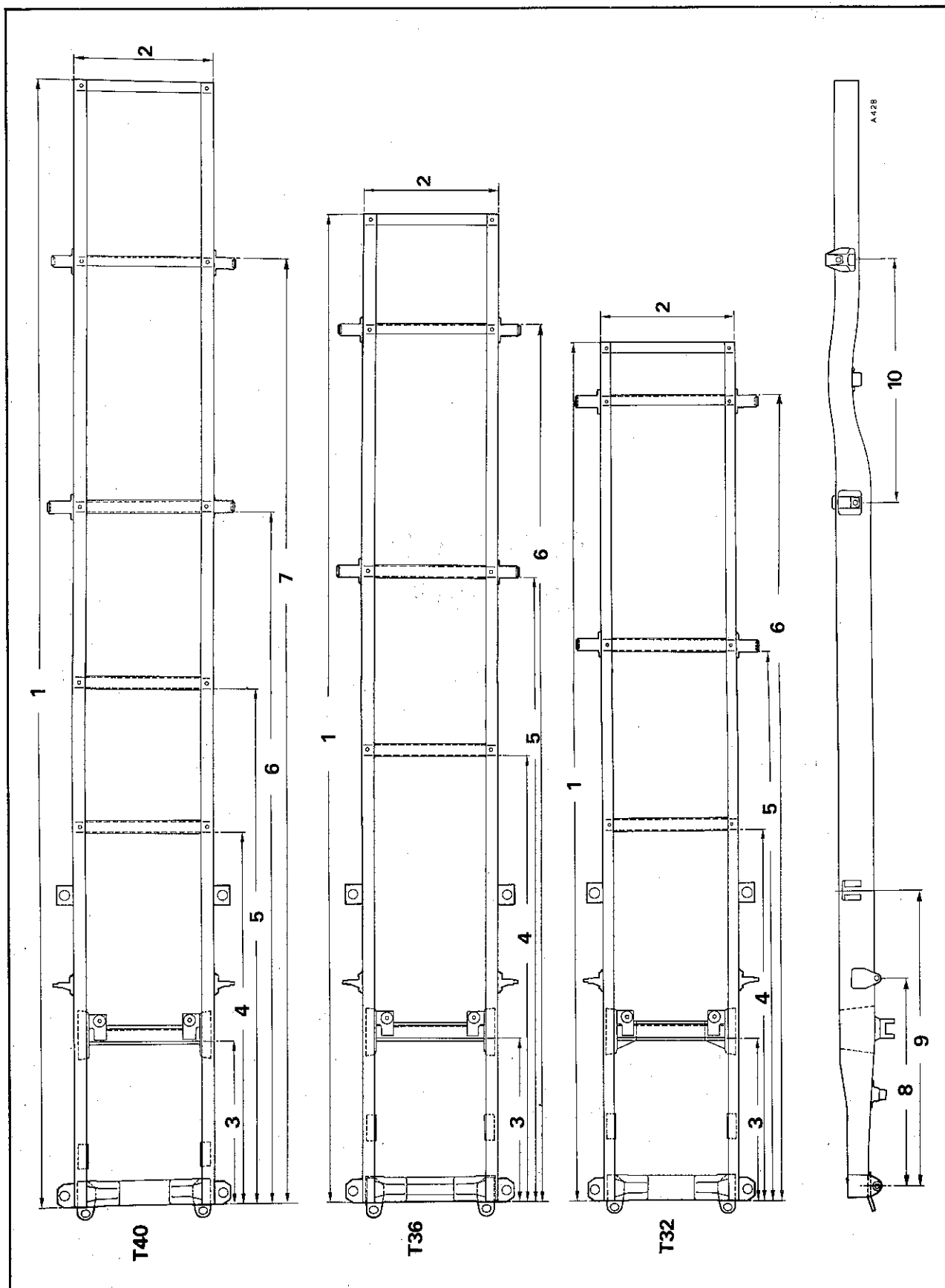
Fig. 1 Frame Dimensions
